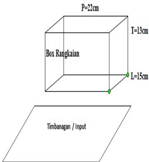
Gambar 5. Rancangan Fisik Alat
