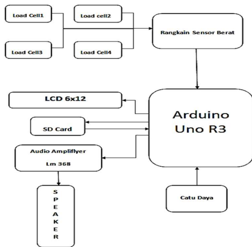
Gambar 2. Blok Diagram Rangkaian
